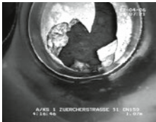
Gebrochene Leitungstücke
