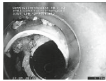
Rohrbruch
