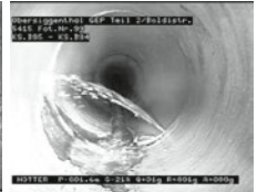
Wassereintritt
